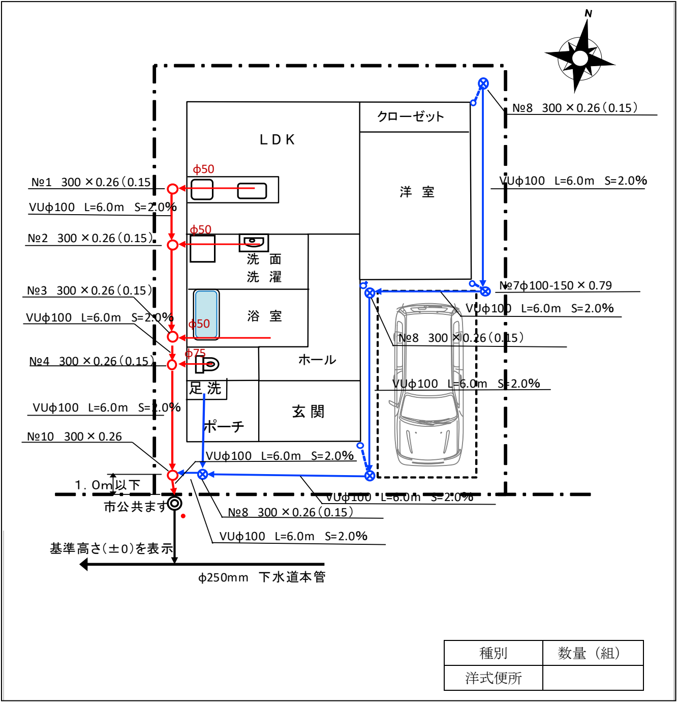
「宅地内分流式使用例」 (参考図)
