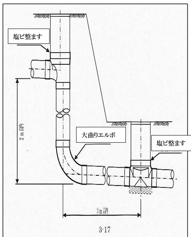
図 3-2 ドロップますの例（硬質塩化ビニル製ます）
