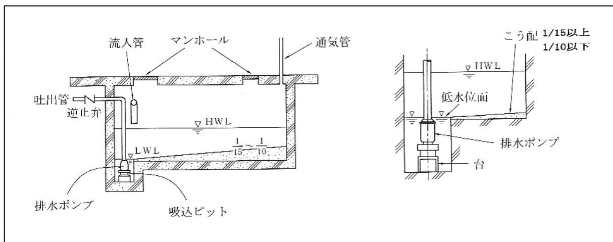
図 2 - 2 排水槽の例
