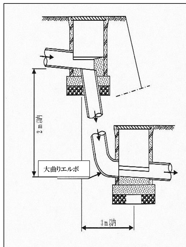
図 3-3 底部有孔ますの例（コンクリート製ます）
