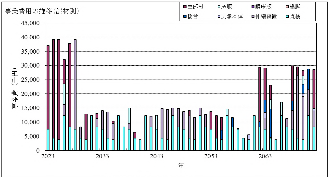
図3-23 部材別事業費の推移
