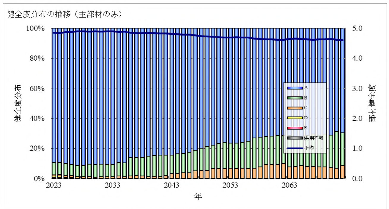
図3-26 主部材別健全度分布の推移
