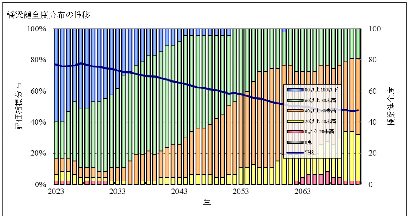
図3-16 橋梁別健全度分布の推移
