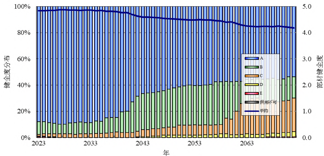
健全度分布の推移（部材別）
