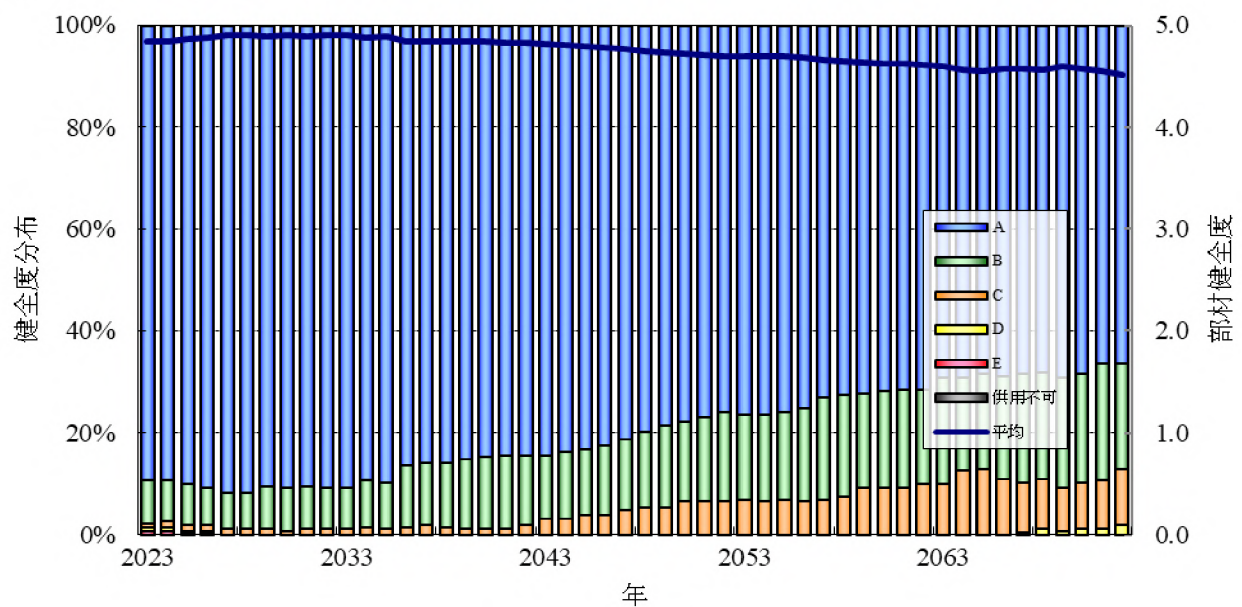
図3-22 主部材別健全度分布の推移
