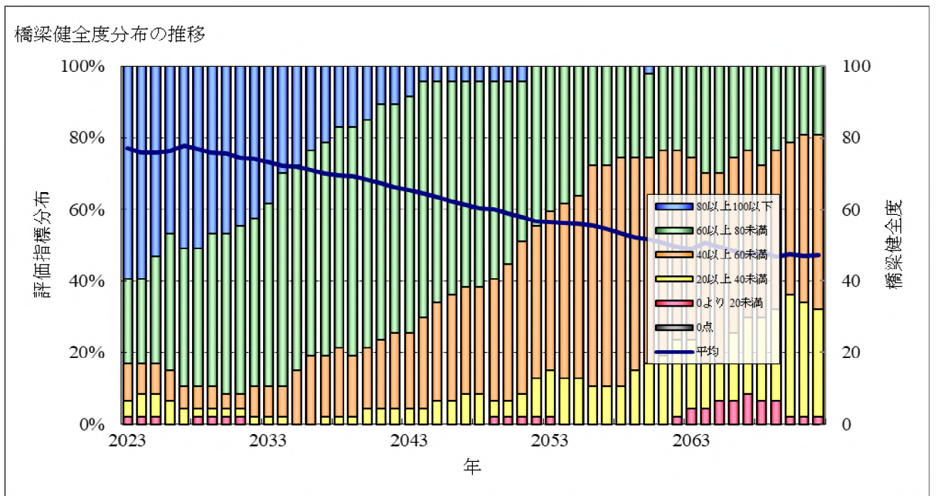
図3-24 橋梁別健全度分布の推移
