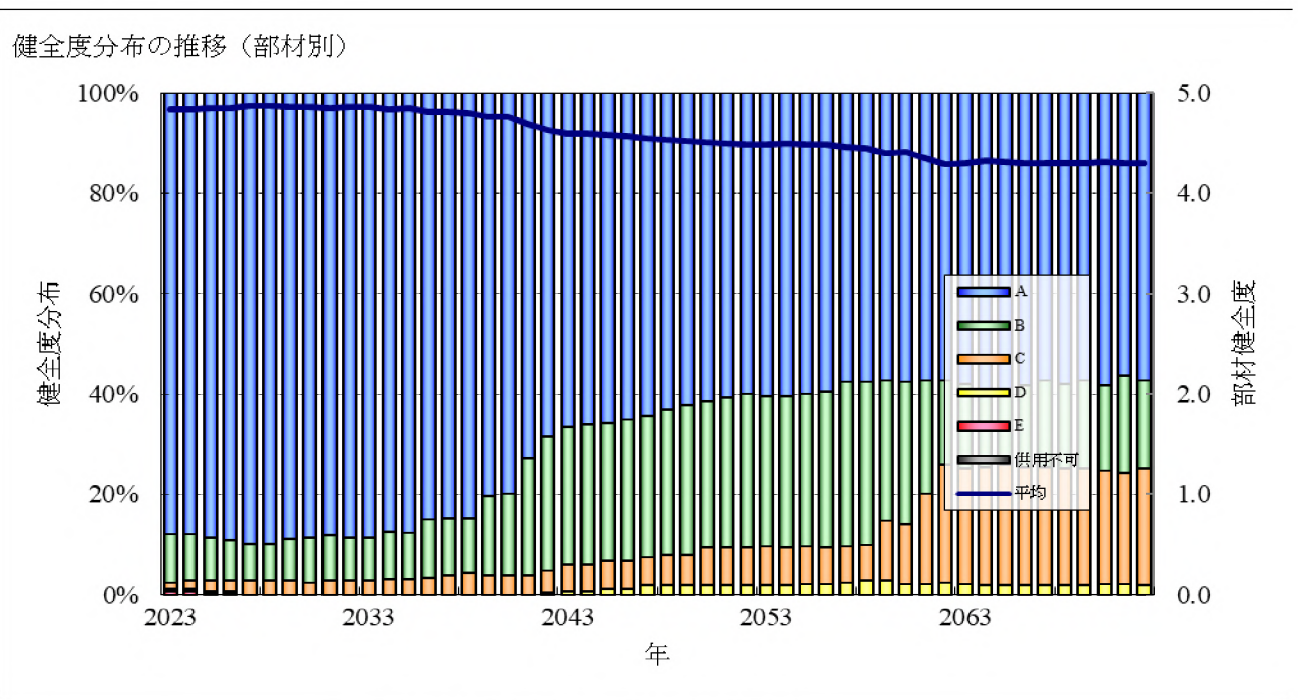
図3-25 部材別健全度分布の推移
