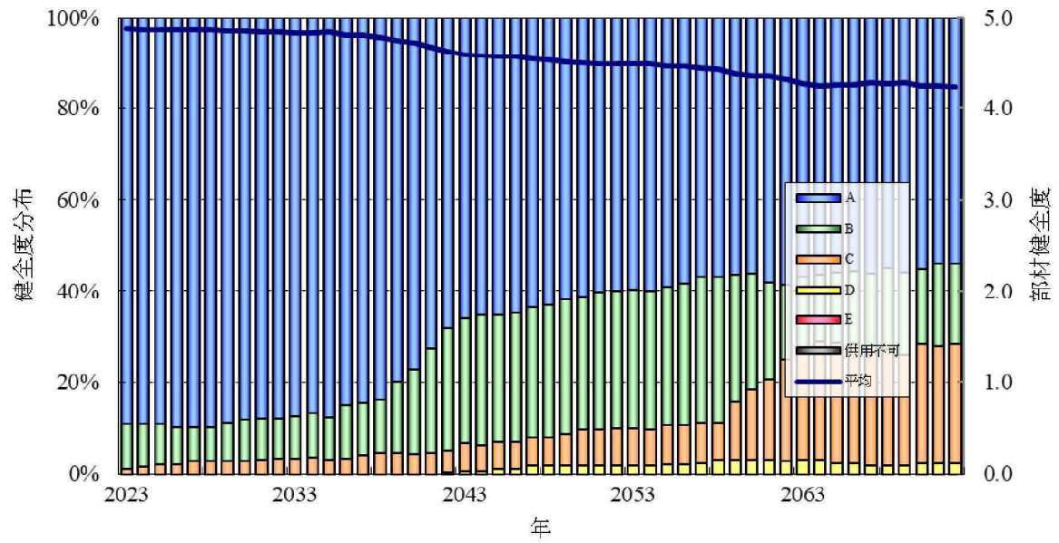
図3-7 部材健全度分布の推移
