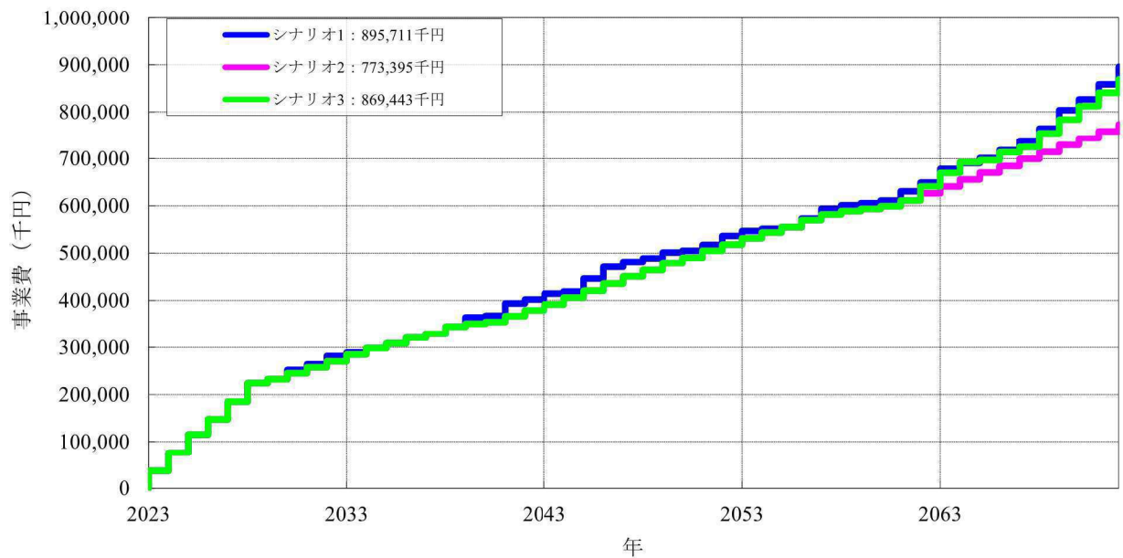
図3-14 累計事業費の比較
