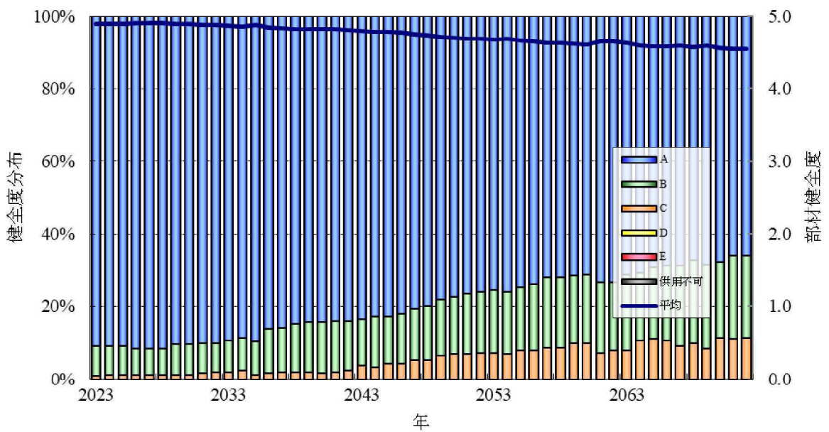
図3-8 主部材健全度分布の推移
