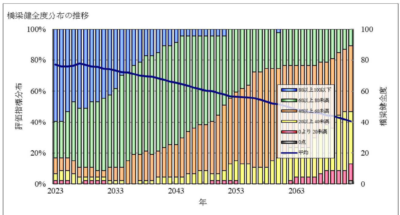
図3-20 橋梁別健全度分布の推移
