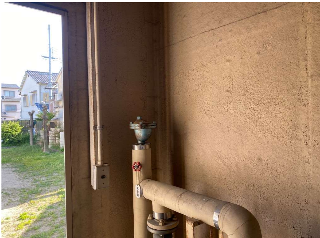
浄化槽写真(その4)
