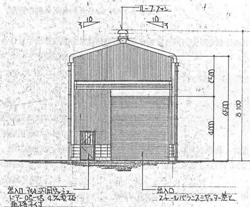
東側立面図 8=100mm
