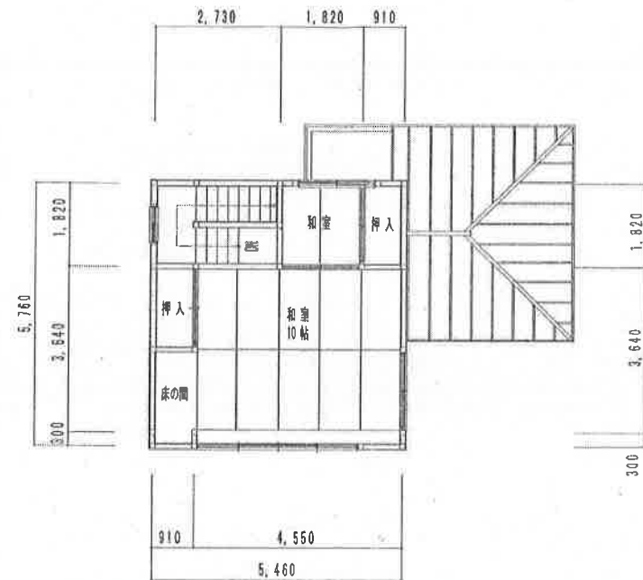
改築2階平面図
