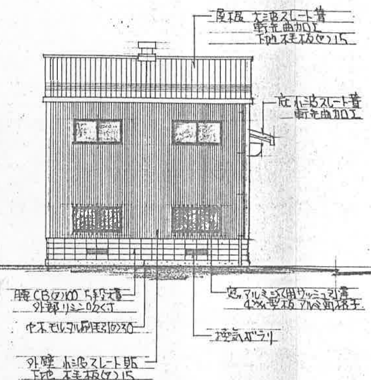
南側立面図 8=100mm
