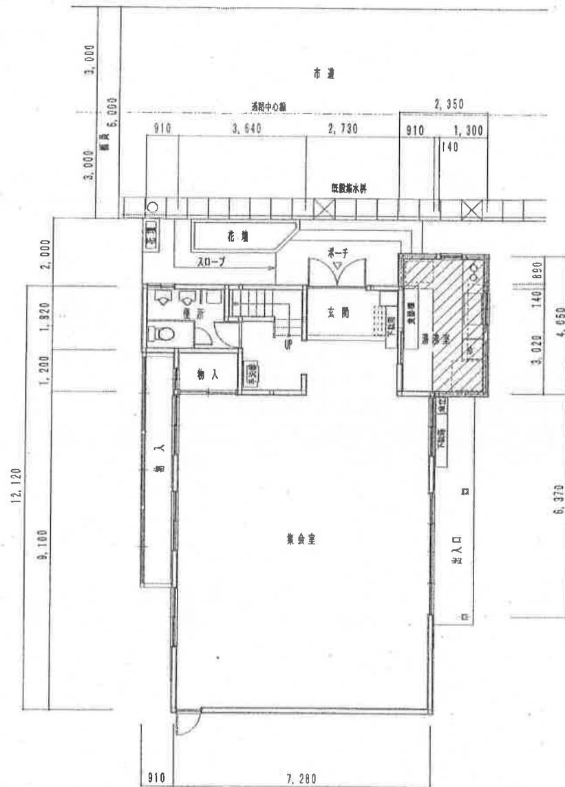
改築1階平面図
