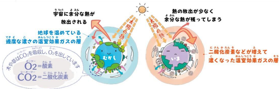
図2-1 地球温暖化の仕組み
