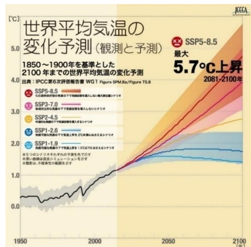
図2-7 世界平均気温の変化予測
