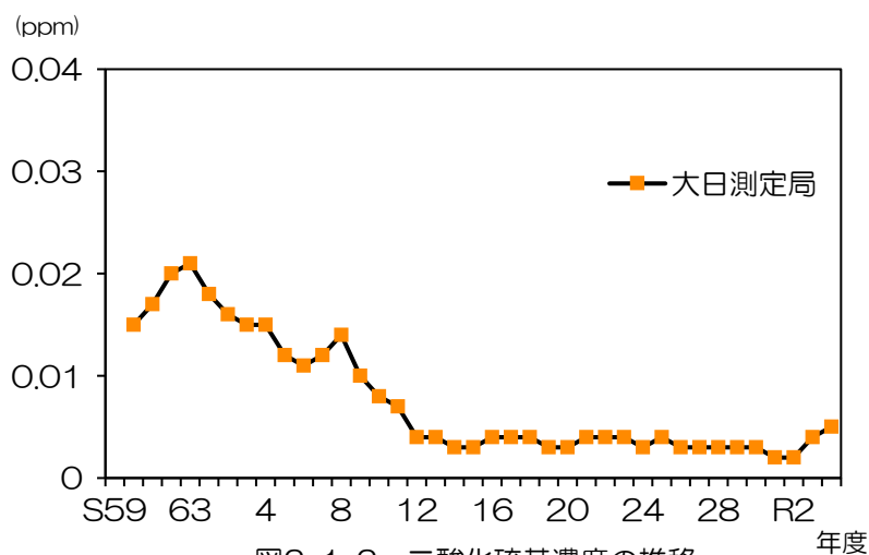
図2-1-2 二酸化硫黄濃度の推移 (1日平均値の2%除外値)
