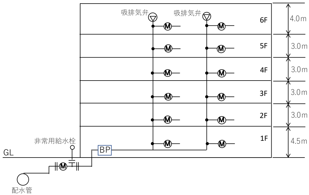
立面図
