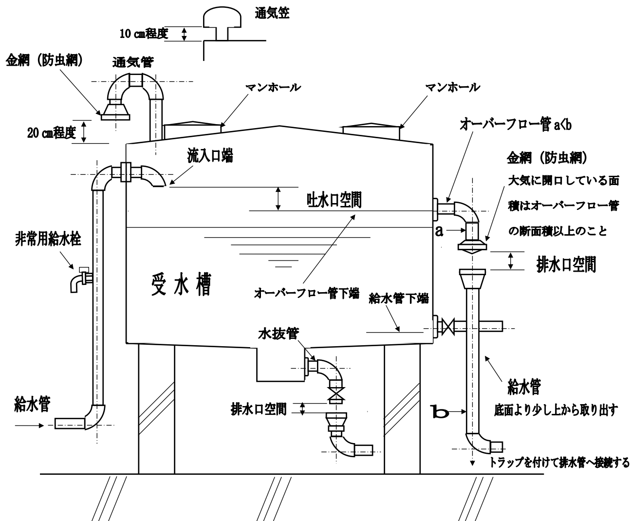
図-10 受水槽などにおける排水口空間等の例
