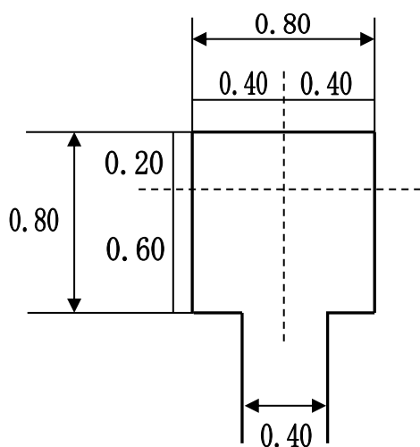
サドル付分水栓取付の場合
