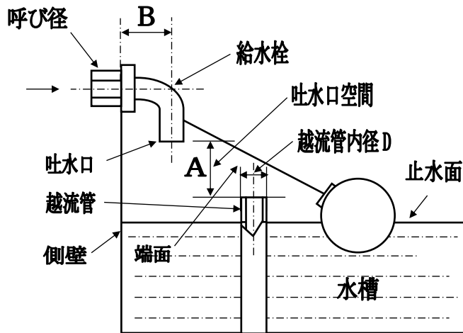
(1) 越流管 (立取出し)
