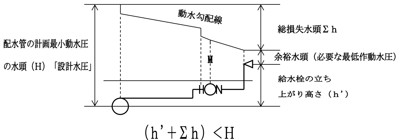
図-3 動水勾配線図
