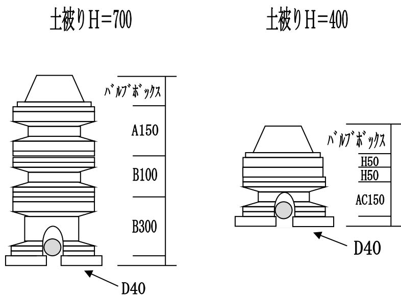
(オ) バルブボックス設置標準図
