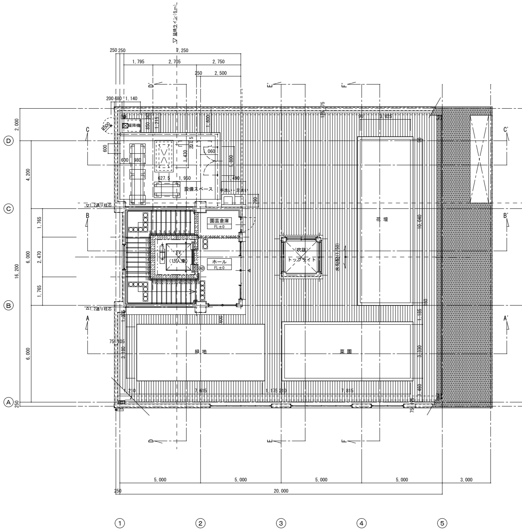
3階 平面図
