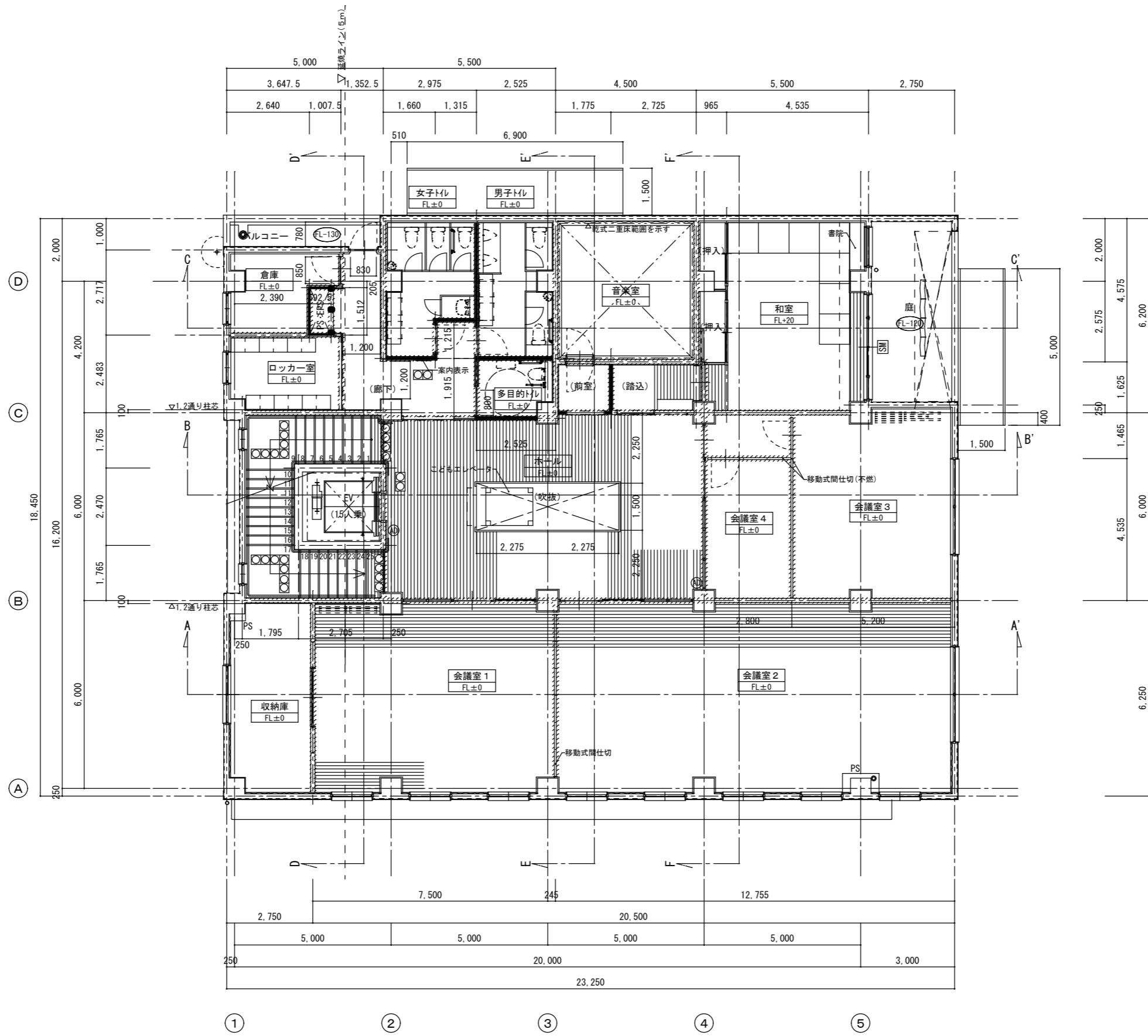
2階 平面図
