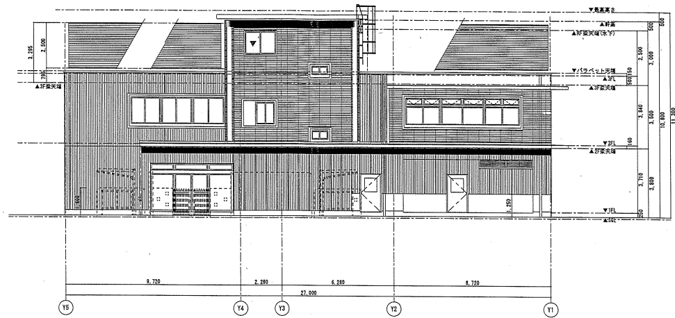
北立面図 S=1/200
