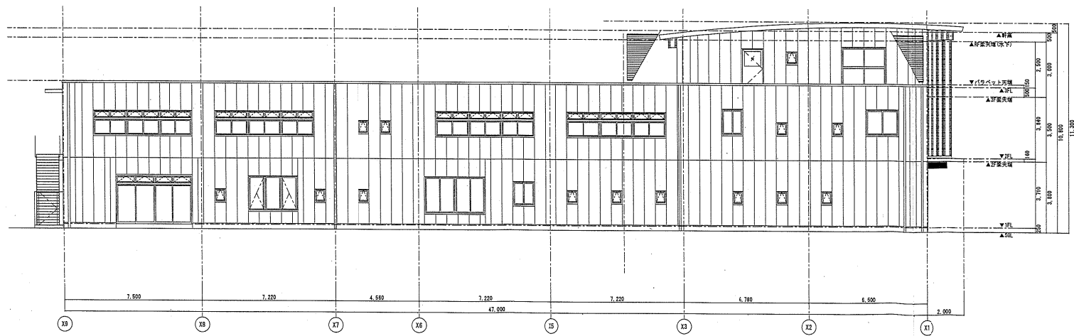
東立面図 S=1/200
