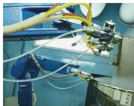
3コート3バイク自動塗装ロボットライン
