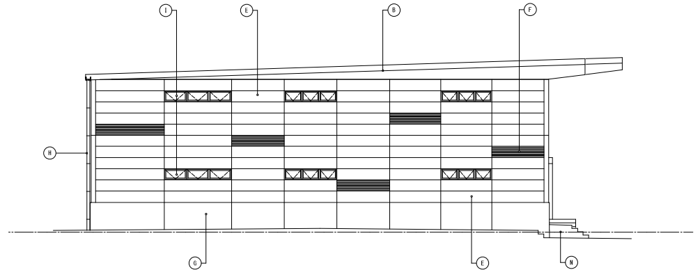
西立面図 1/200
