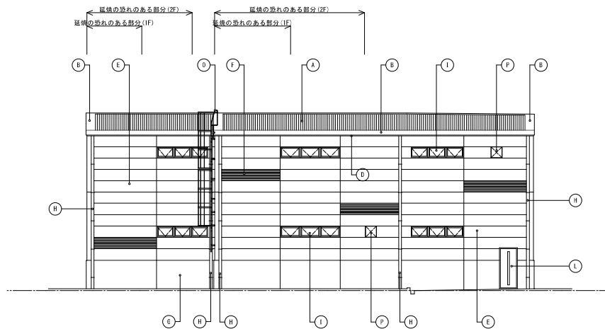
北立面図 1/200
