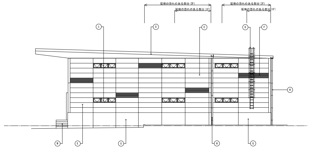
東立面図 1/200
