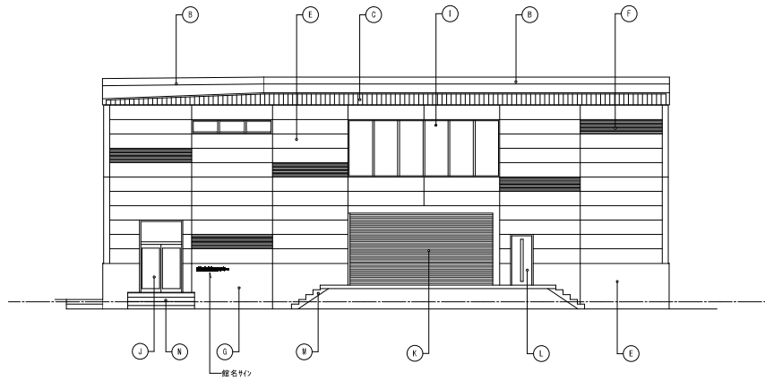
南立面図 1/200
