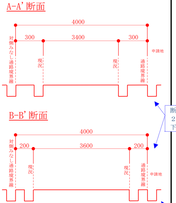
(通路断面) 2ヶ所
