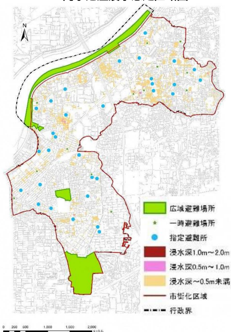
内水氾濫浸水想定区域図
