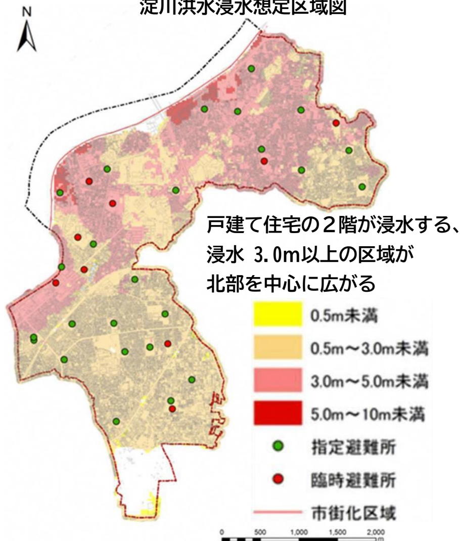
淀川洪水浸水想定区域図
